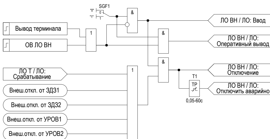
Рисунок 2.16 – Функциональная схема ЛО ВН
